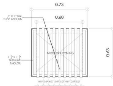
ELEVATION "C"
